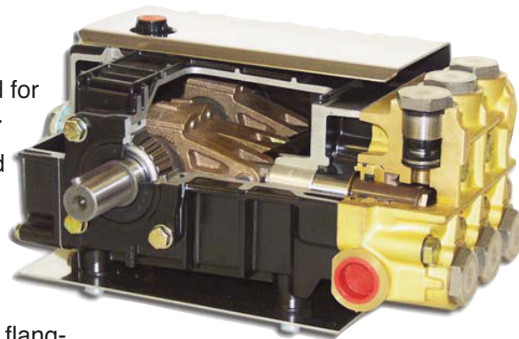
Schnittmodell der typischen Reihenkolben-Hochdruckpumpe
